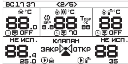
Экран №2 «Контуры отопления»
