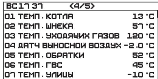
Экран №4 «Датчики»
